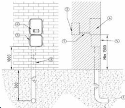
Figura 5: Acometida subterránea en fachada, distancias expresadas en mm.
