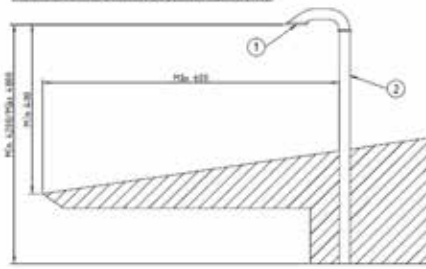
Figura 3. Distancias en aleros en mm.
