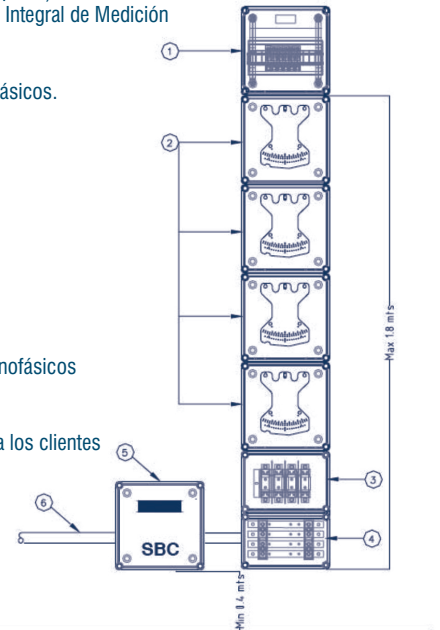
b) Disposición de las columnas que componen el Gabinete Integral de Medición
