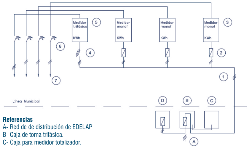
a) Esquema eléctrico para acometidas en Gabinetes Integrados de Medición Figura 1. Esquema de conexión eléctrica para suministros monofásicos y trifásicos
