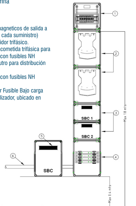
Figura 4. Acometidas en Gabinetes Individuales
