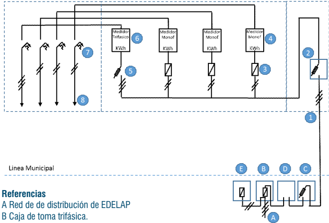
Figura 1. Esquema de conexión eléctrica para suministros monofásicos y trifásicos
